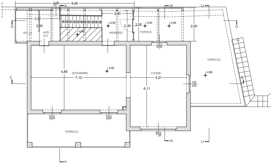
STATO DI PROGETTO PIANTA PIANO SOTTOTETTO
